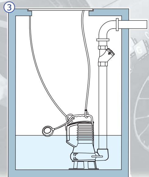
Instalación fija mediante tubo metálico roscado
