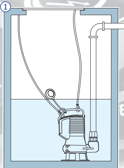
Instalación mediante tubo y relativo racor de polietileno
